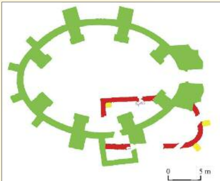
Pôdorys rímskokatolíckeho Kostola sv. Kozmu a Damiána. Zelená farba – barokový kostol, červená farba – starší, zrejme románsky kostol, žltá farba – stavebné úpravy pôvodného kostolíka.
