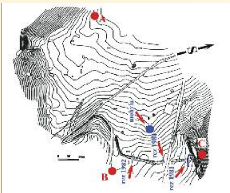
Geodetický plán hradiska Pri dúbravskej studničke s priebehom valu a miestami nálezov.
