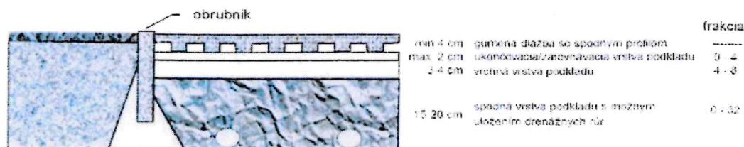
Obr.3 Hĺbkový profil osadenia gumovej dlažby.
